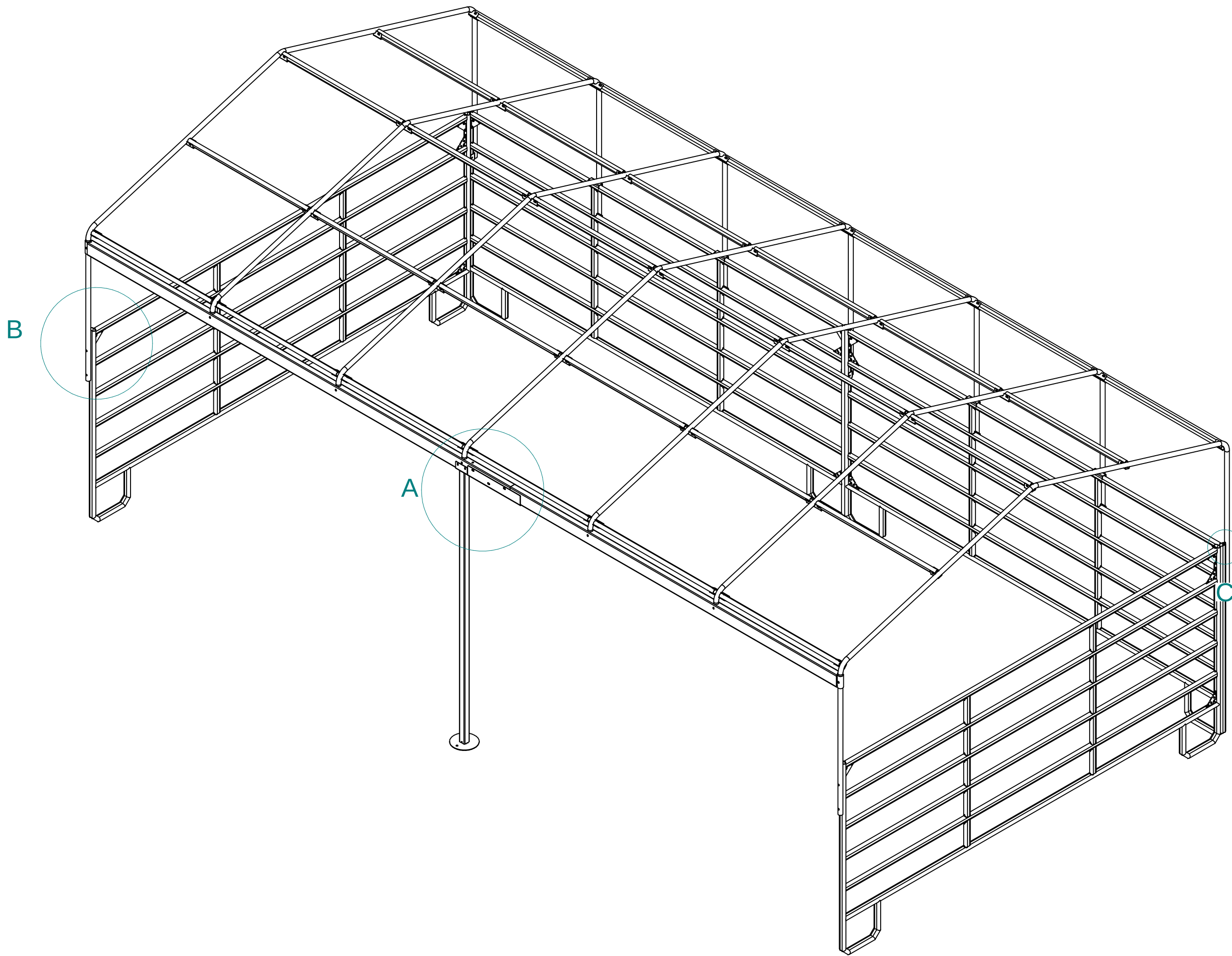
přístřešek 3,6x7,2m
